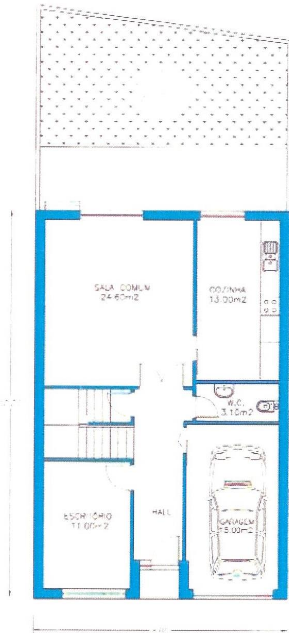
PLANTA DO TÉRREO
