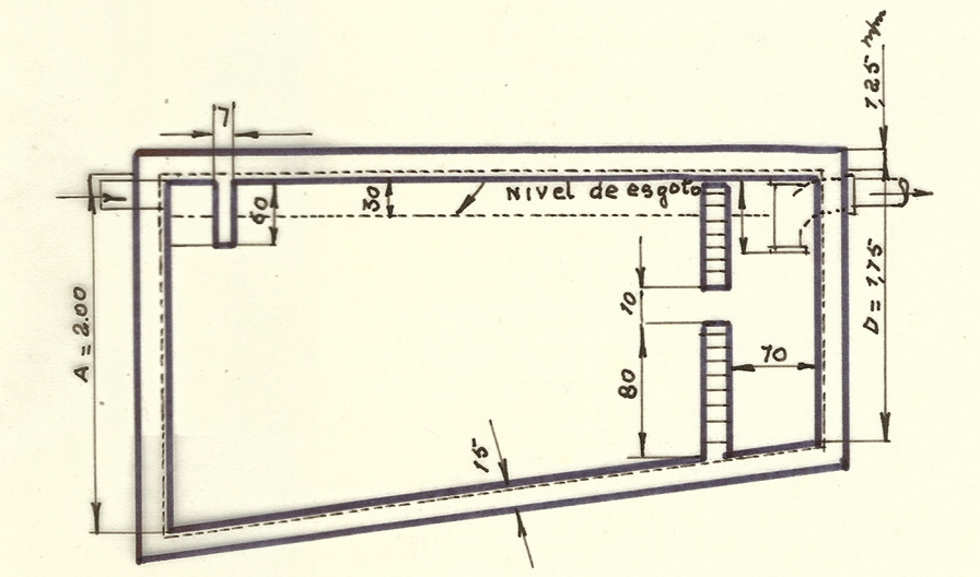
corte b-b
