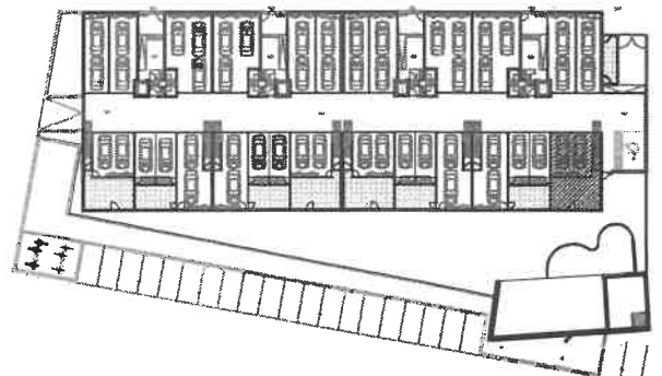
PISO 0
