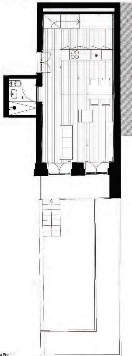
Planta Piso 1
