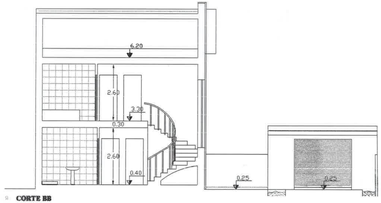
CORTE BB
