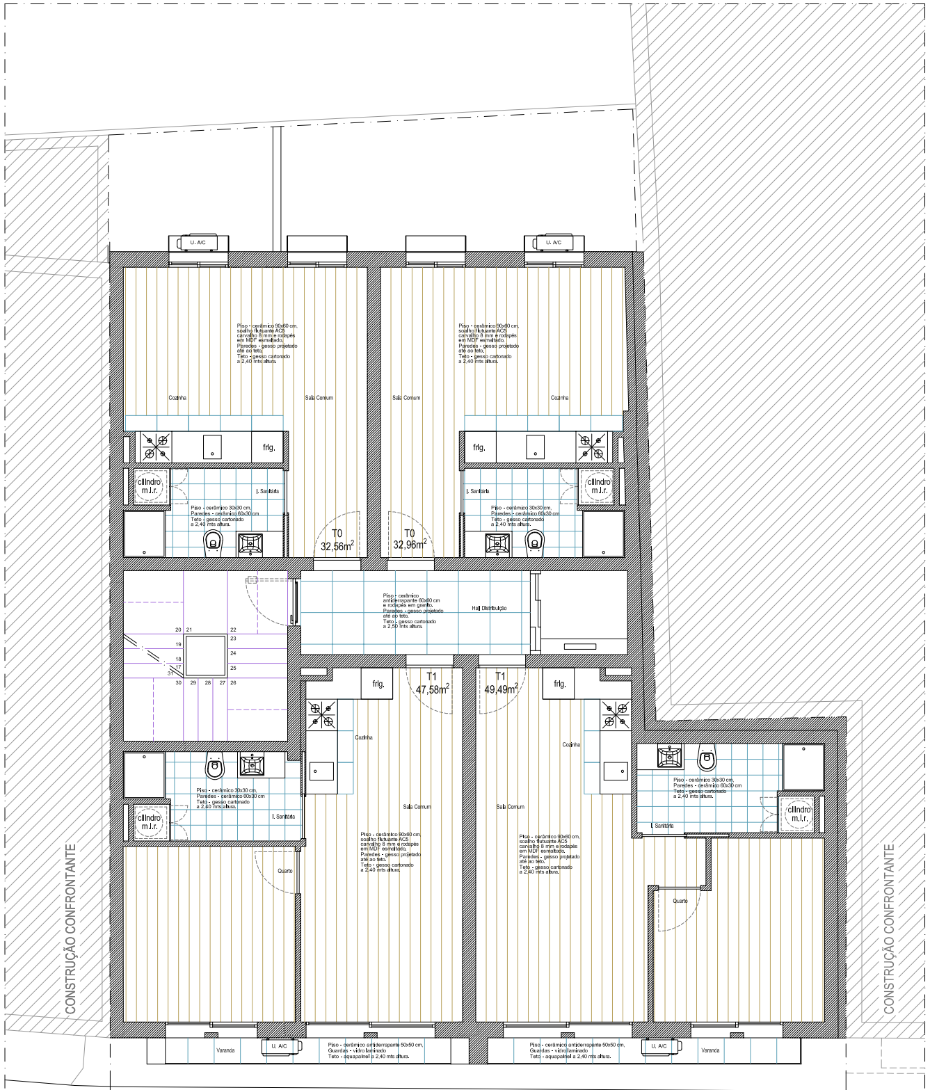
PLANTA DO PISO 1 / 2 / 3
