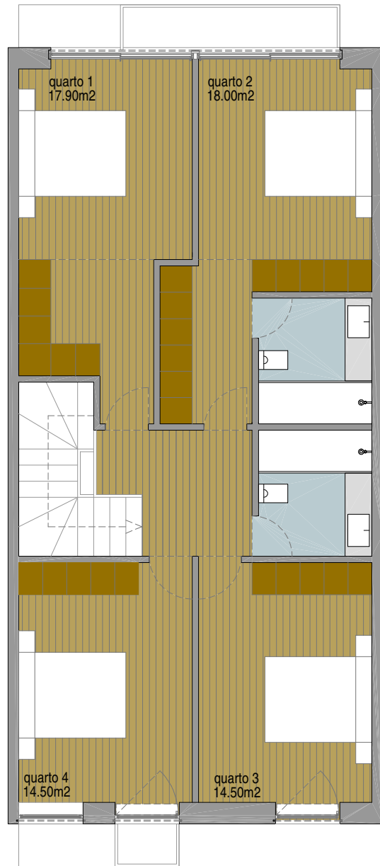
PLANTA DO ANDAR
