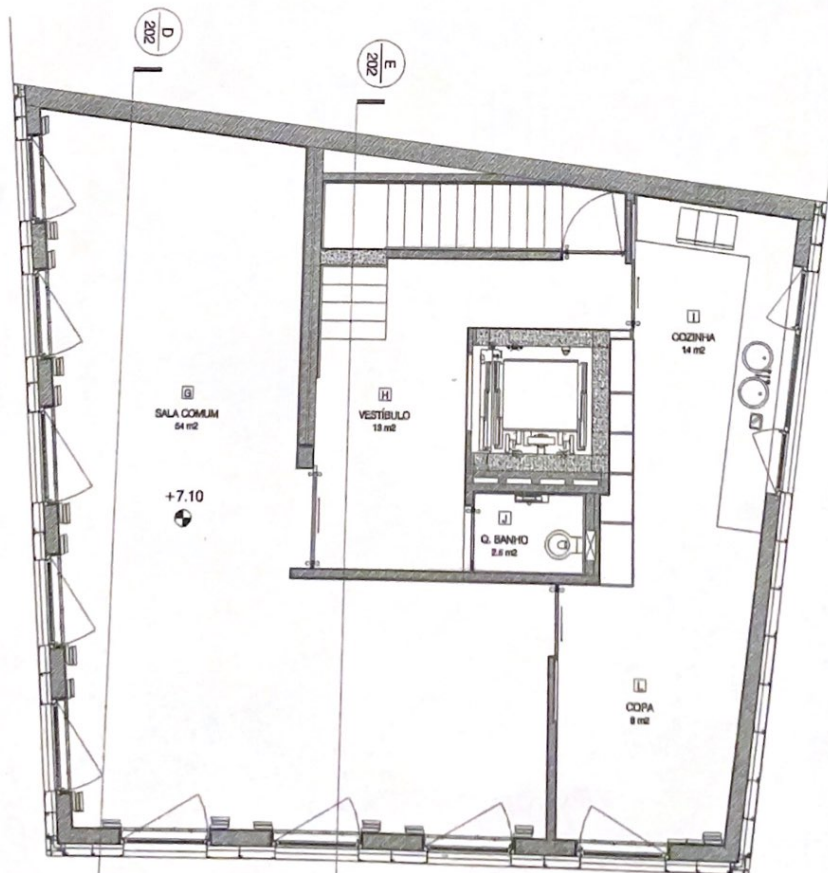
D. PLANTA PISO 2
