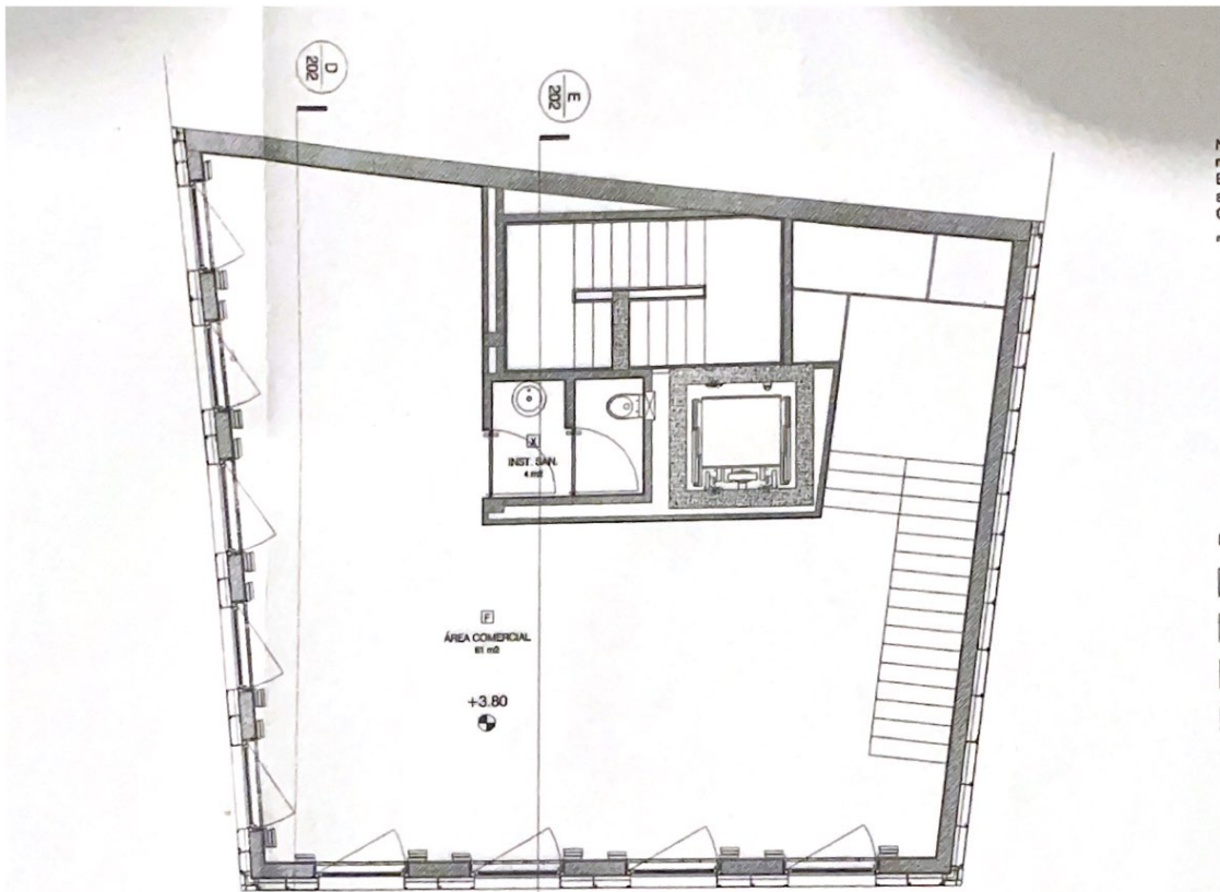
C. PLANTA PISO 1
