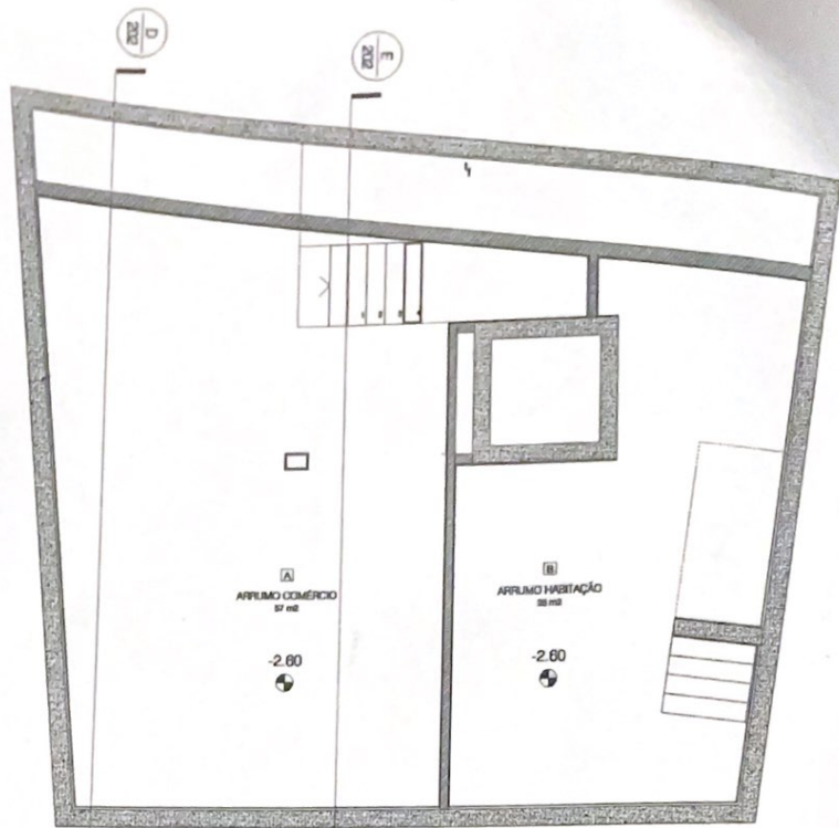
A. PLANTA PISO -1
