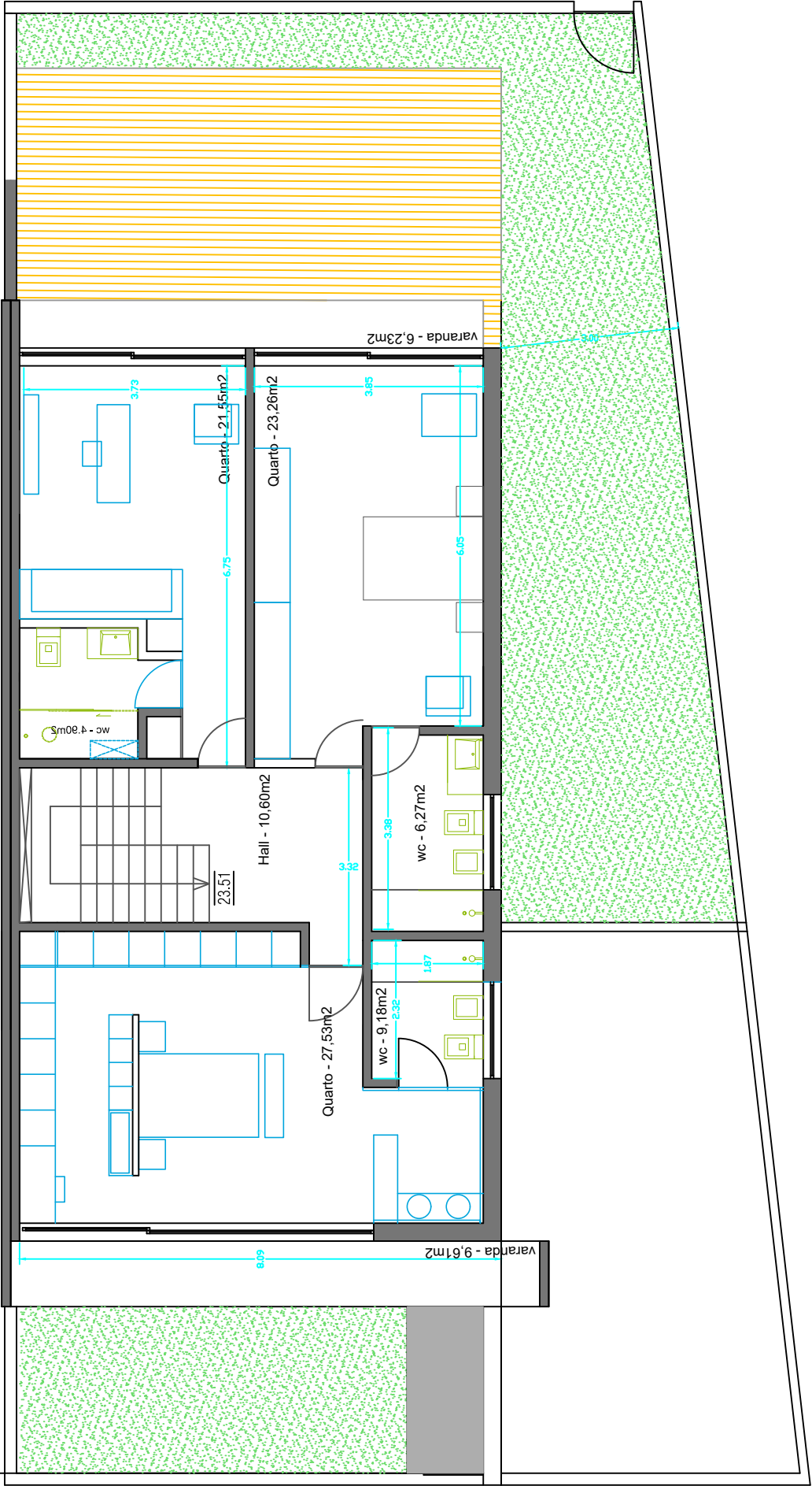
Planta Piso 1
