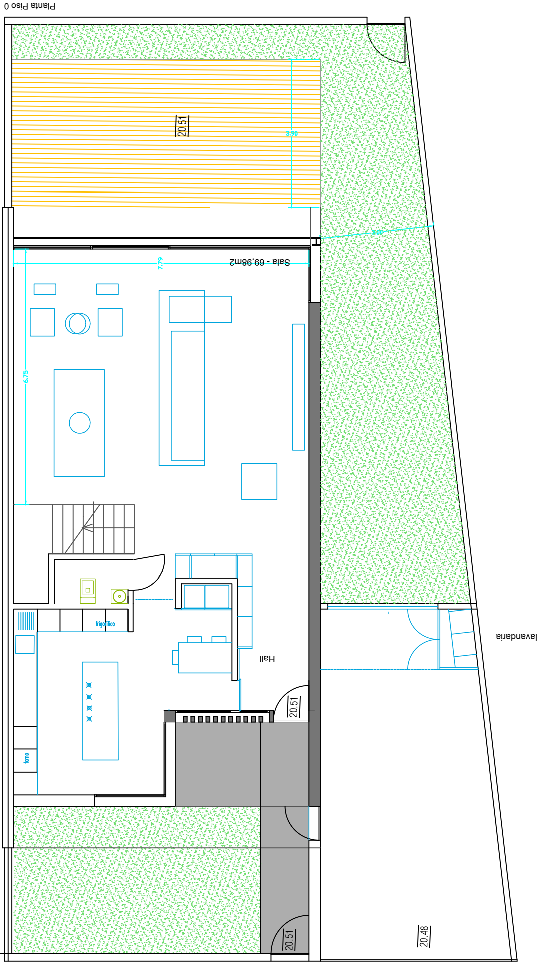
Planta Piso 0
