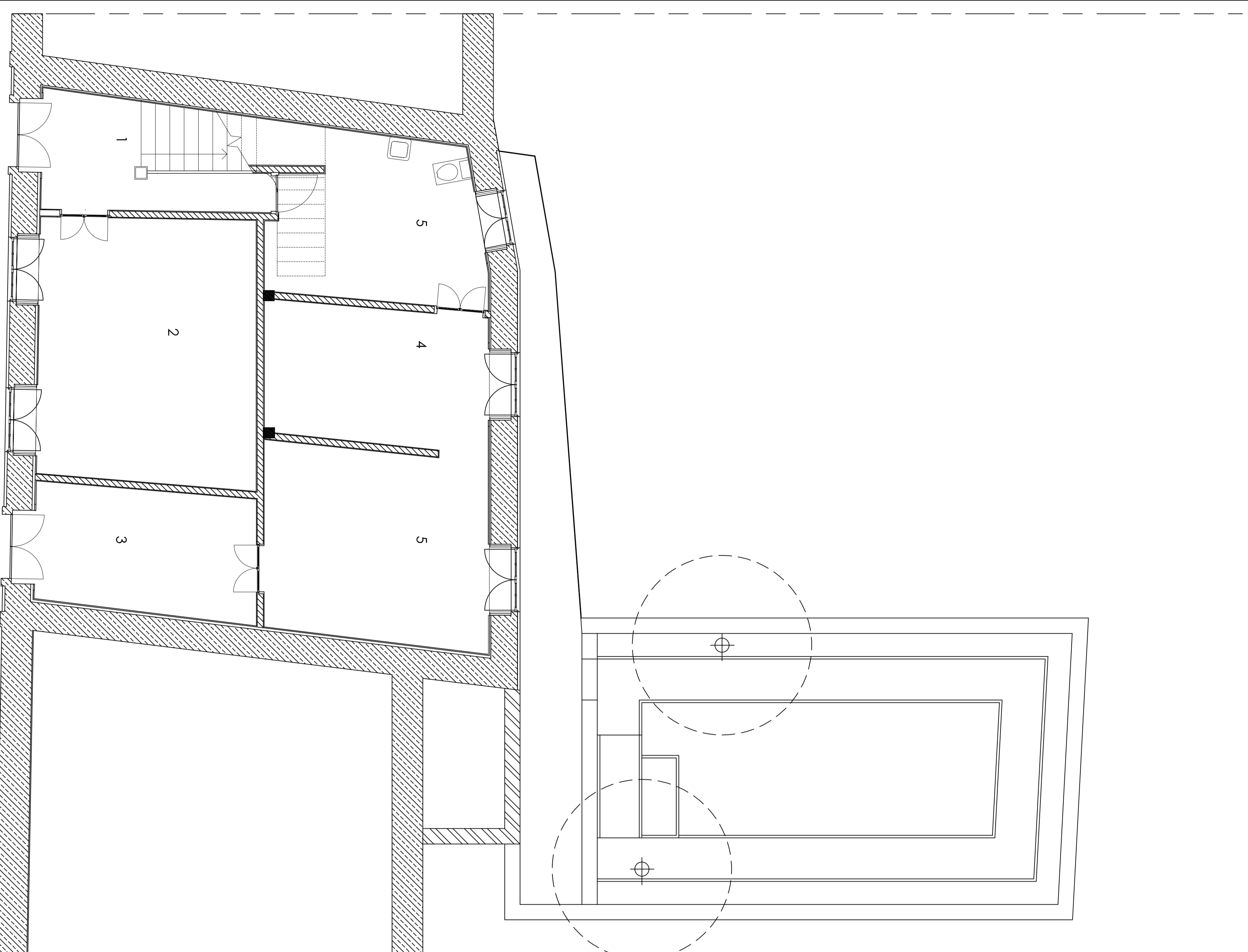
Planta Rés do Chão
