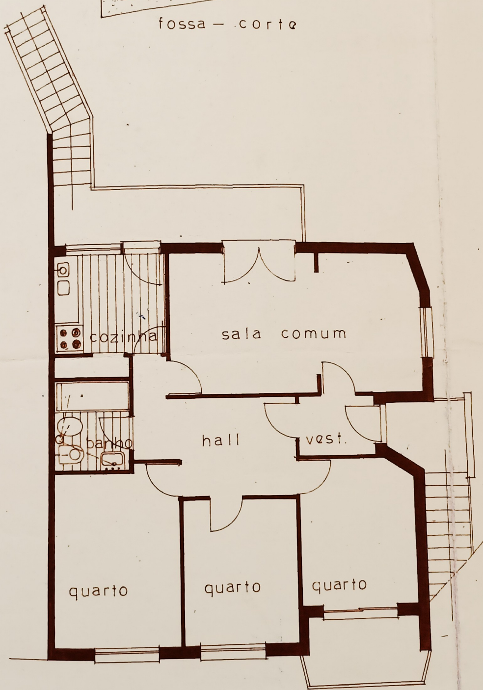
PLANTA DO ANDAR
