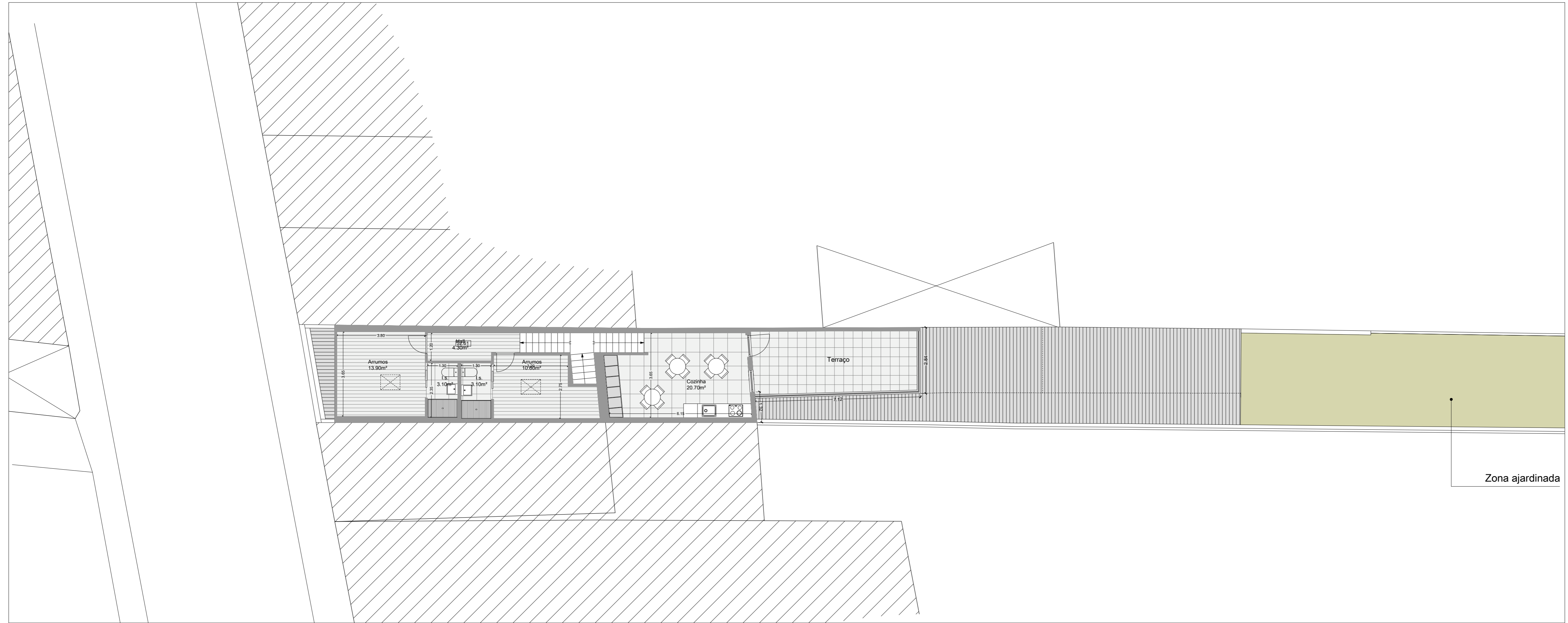
PLANTA DO ANDAR
